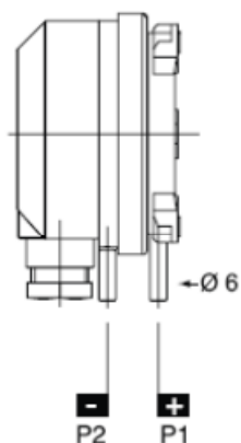
Obr.: Pripojenie snímača tlakových rozdielov
